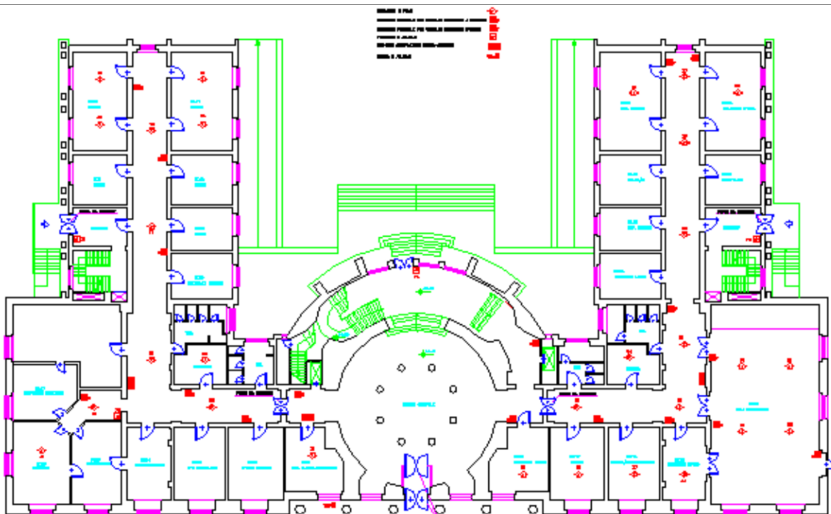
Figura 2 - Piano terra edificio principale
