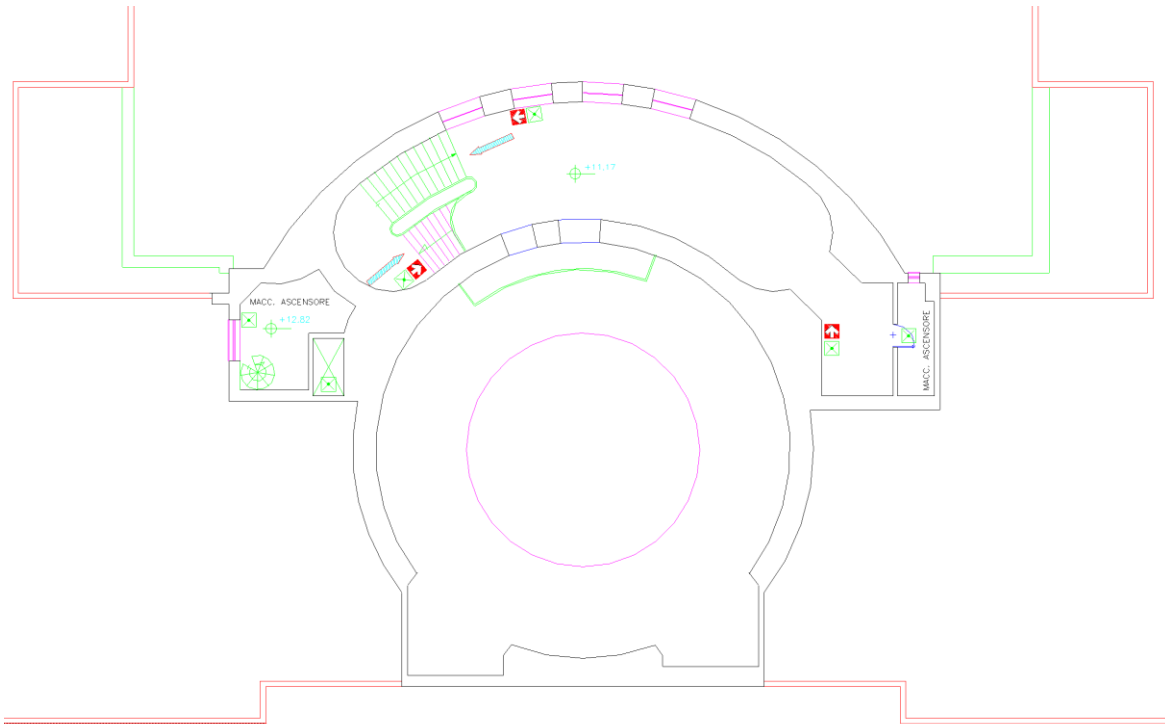
Figura 5 - Piano terzo edificio principale
