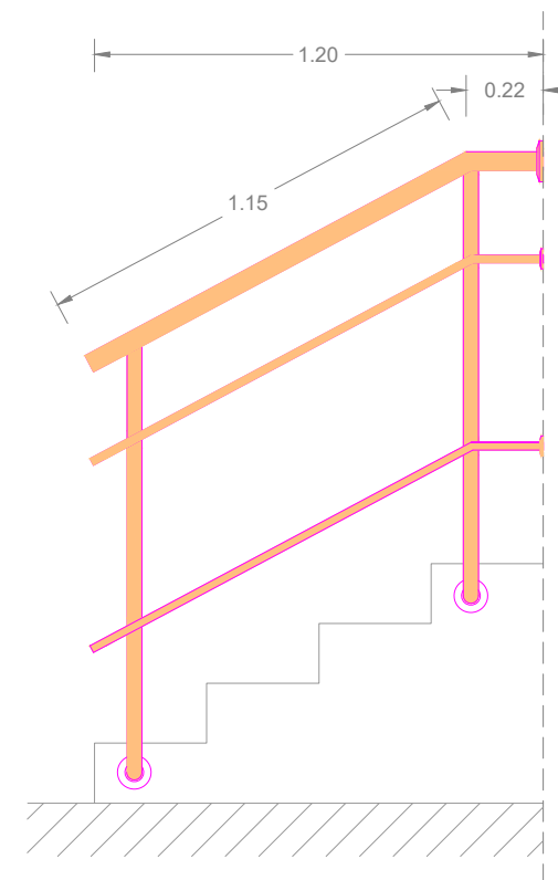
DETTAGLIO RINGHIERA SCALE scala 1:20
