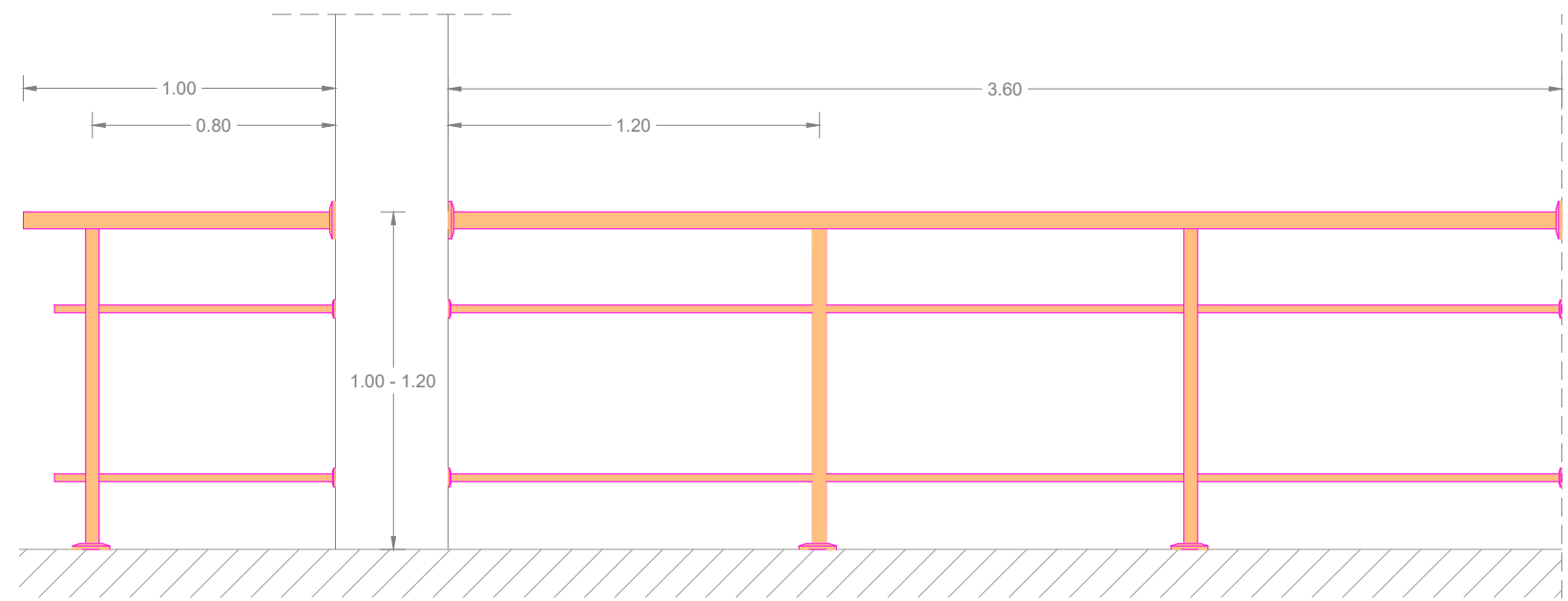
DETTAGLIO RINGHIERA scala 1:20
