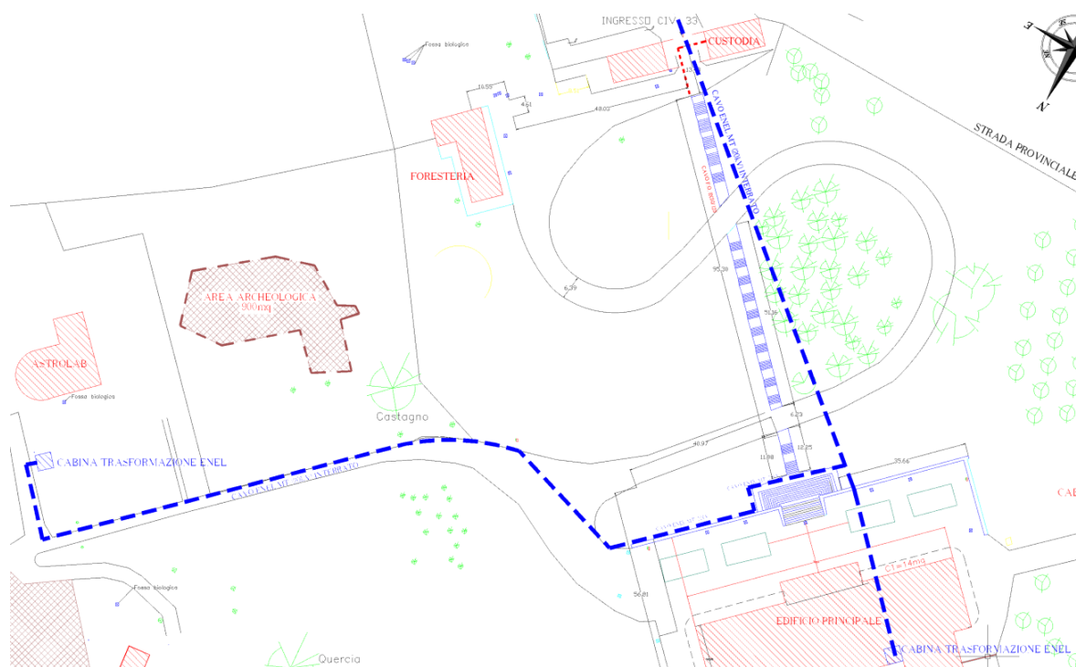
Figura 8 - passaggio delle linee elettriche dell'ENEL a media tensione (20.000V) e indicazione delle cabine di trasformazione da 20.000 Volt
